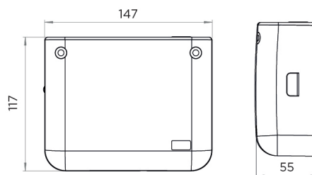
Dimensiones (mm)
